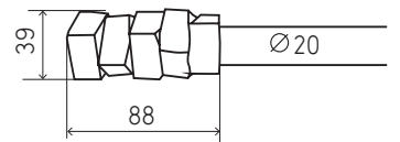
EMBOUT FRAGILE 20
