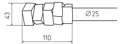
EMBOUT FRAGILE 25
